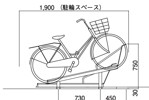
側面図
