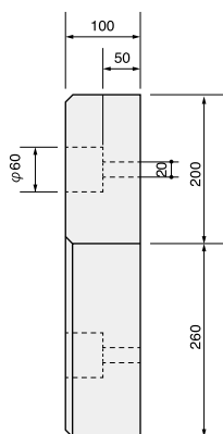
FWGH-1046（無垢）
