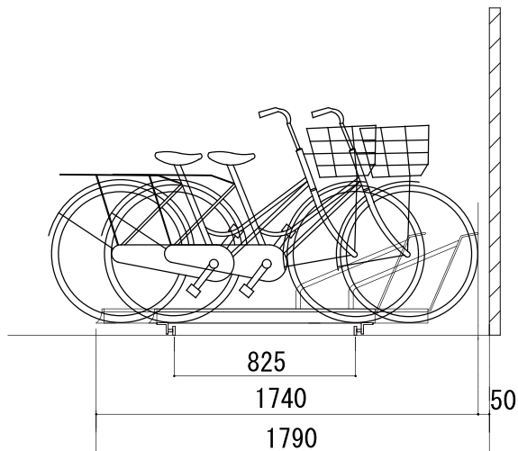
側面図
